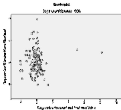
Gambar 3 Uji Heteroskedastisitas
